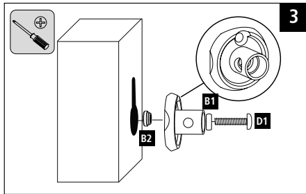
Installation with key hole Montage bei Schlüssellochabhängung
