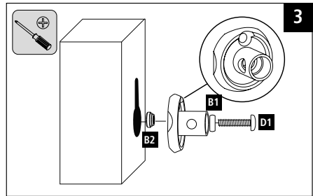
Installation with key hole Montage bei Schlüssellochabhängung
