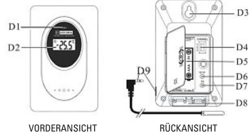
VORDERANSICHT
